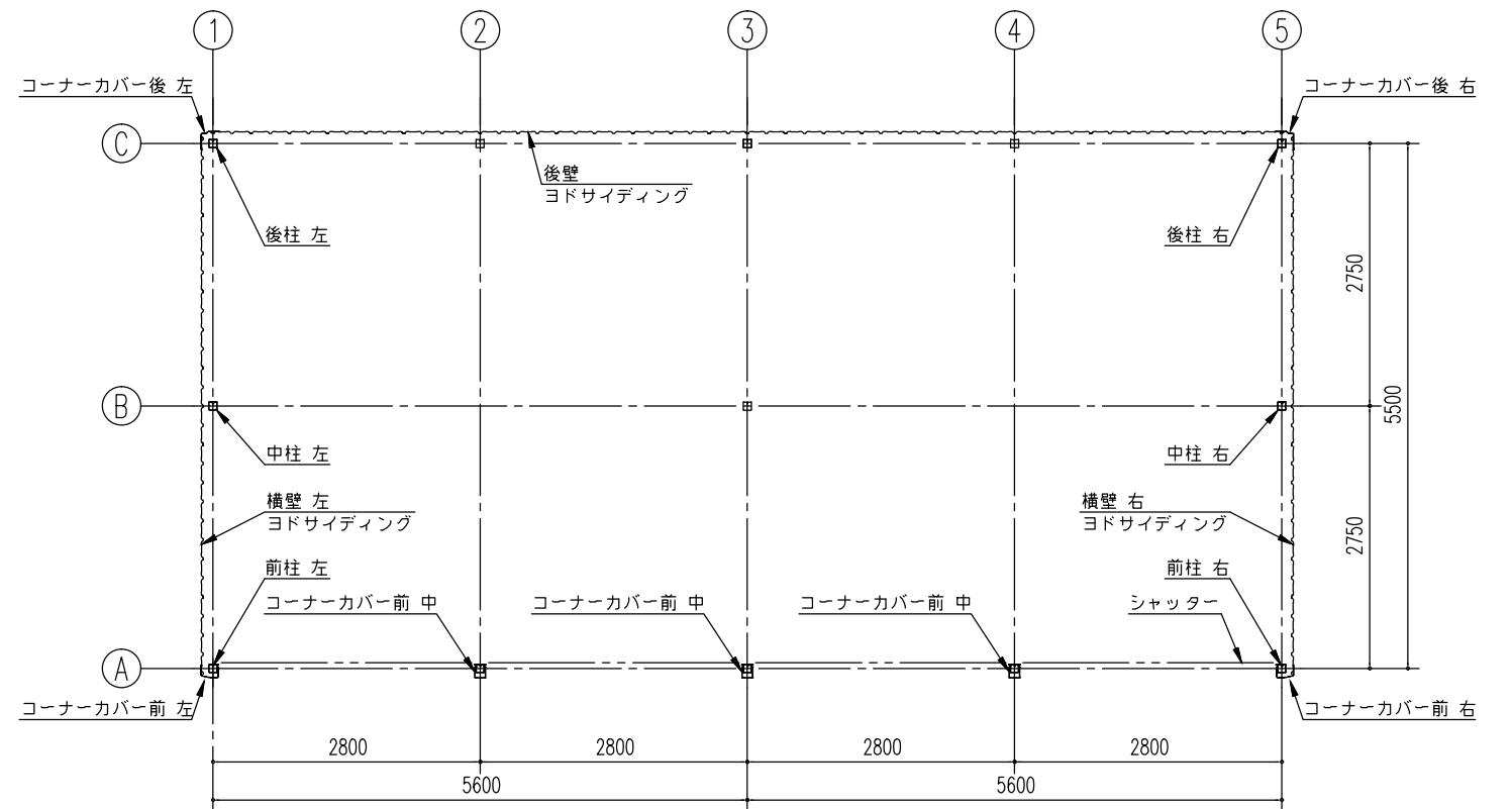
平面図 (S=1/80)
