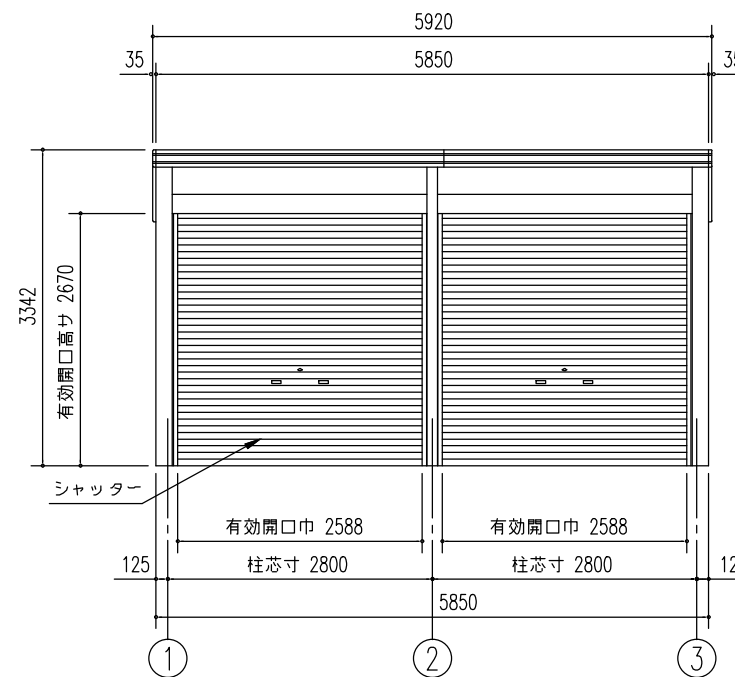
正面立面図(S=1/80)
