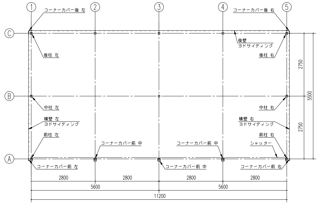
平面図 (S=1/80)
