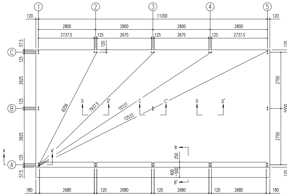
基礎伏図 (S=1/80)
