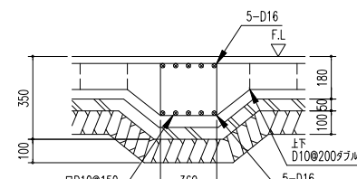
D ~ D' 断面
