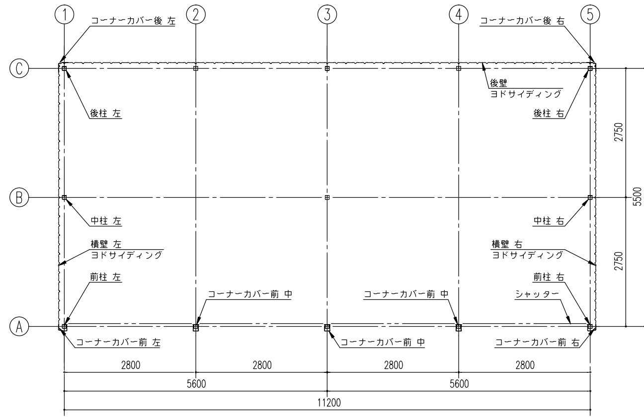
平面図 (S=1/80)
