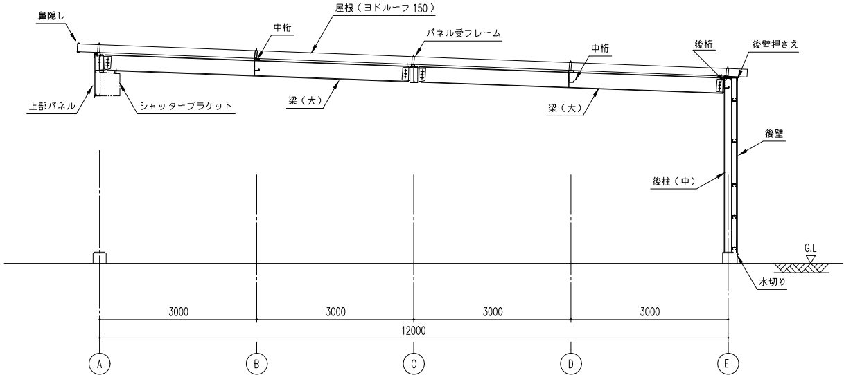
矩 計 図 (S=1/50)
