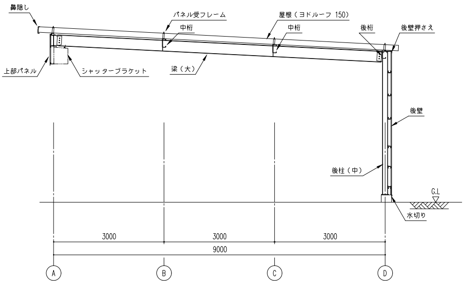
矩 計 図 (S=1/50)
