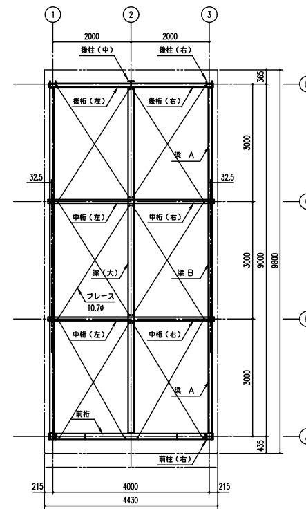
小屋伏図 (S=1/50)
