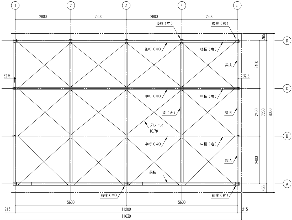
小 屋 伏 図 (S=1/50)
