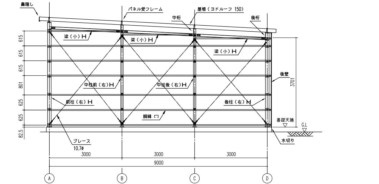
側面断面図 (S= 1/50)
