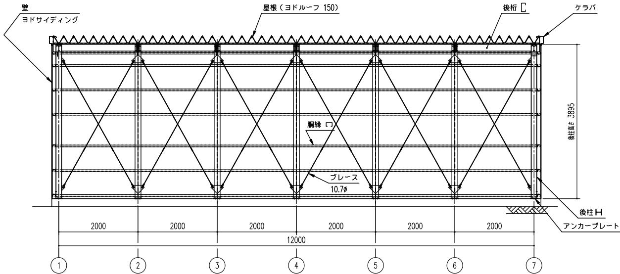
正面断面図 (S= 1/50)
