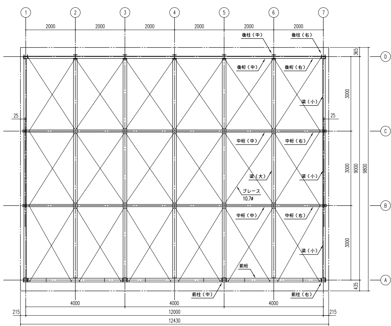
小 屋 伏 図 (S=1/50)
