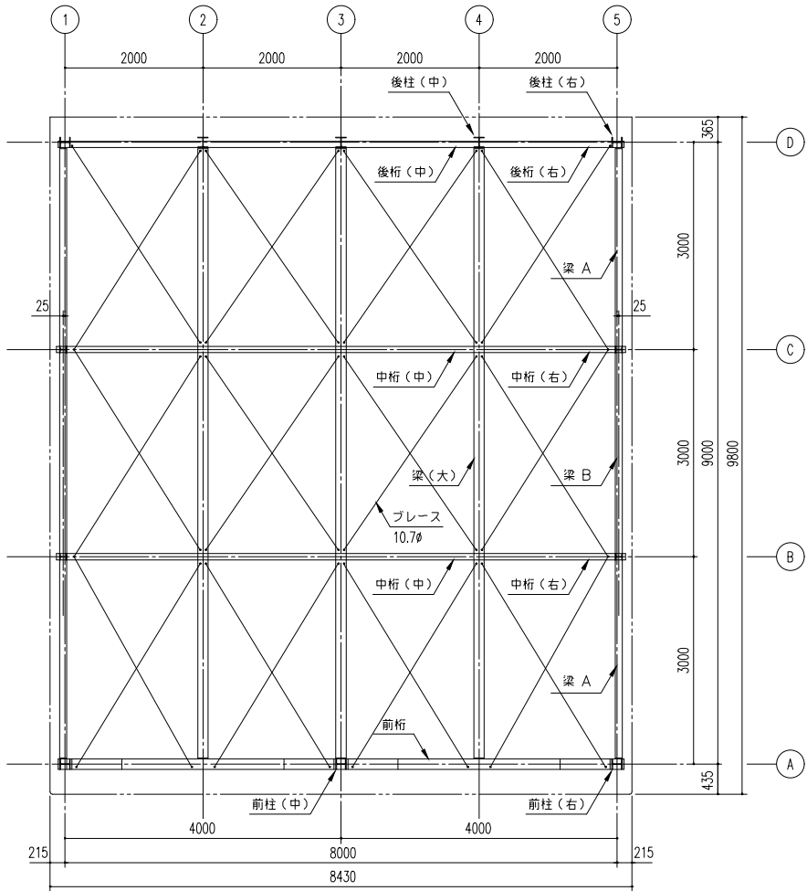
小 屋 伏 図 (S=1/50)
