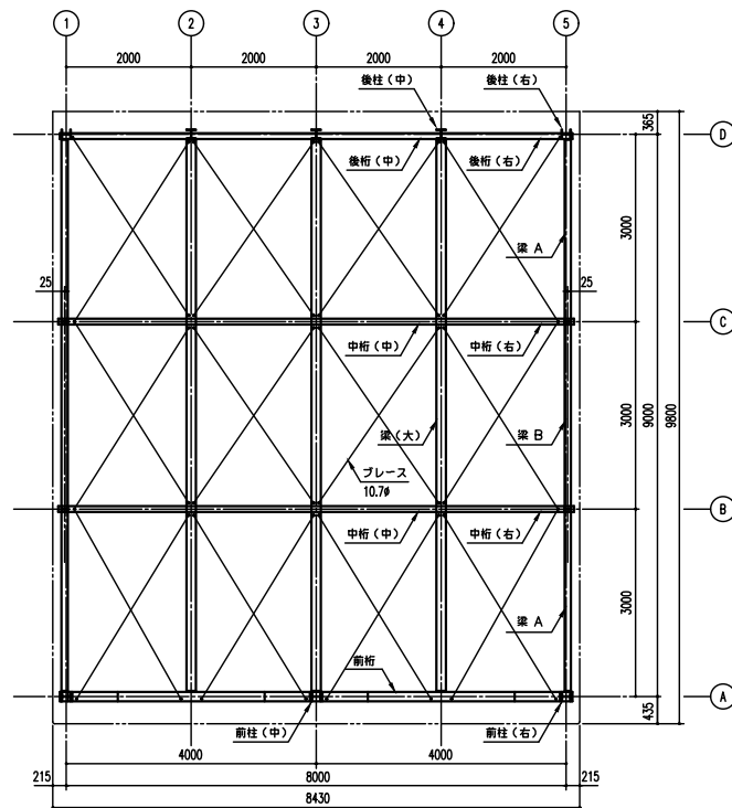
小屋伏図 (S=1/50)
