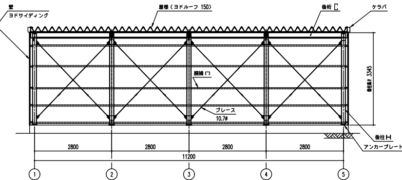
正面断面図 (S=1/50)
