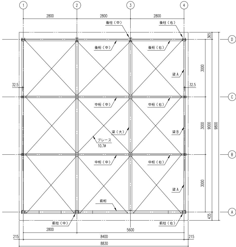
小 屋 伏 図 (S=1/50)
