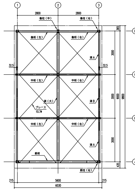
小屋伏図 (S=1/50)
