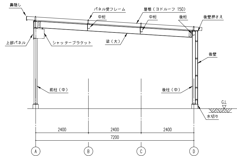
矩 計 図 (S=1/50)
