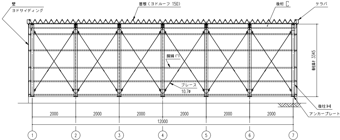
正面断面図 (S= 1/50)
