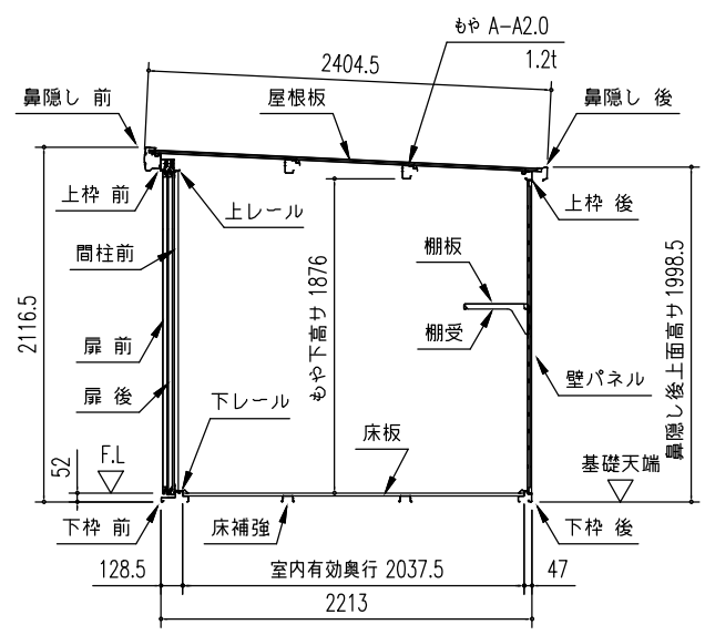
短計図 (S = 1/50)
