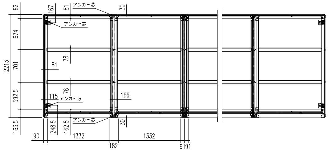
床伏図 (S = 1/50)
