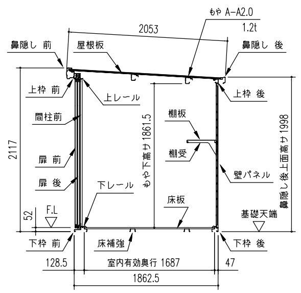
短計図 (S = 1/50)
