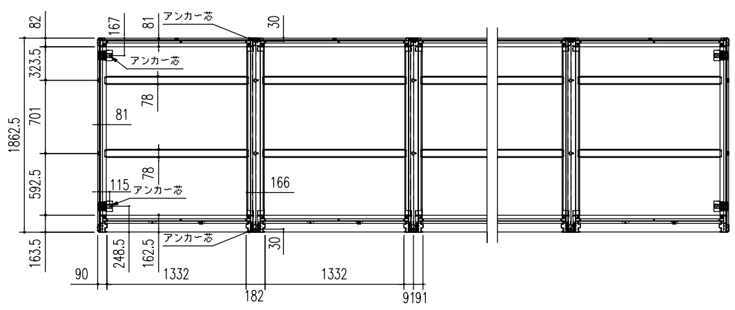
床伏図 (S = 1/50)
