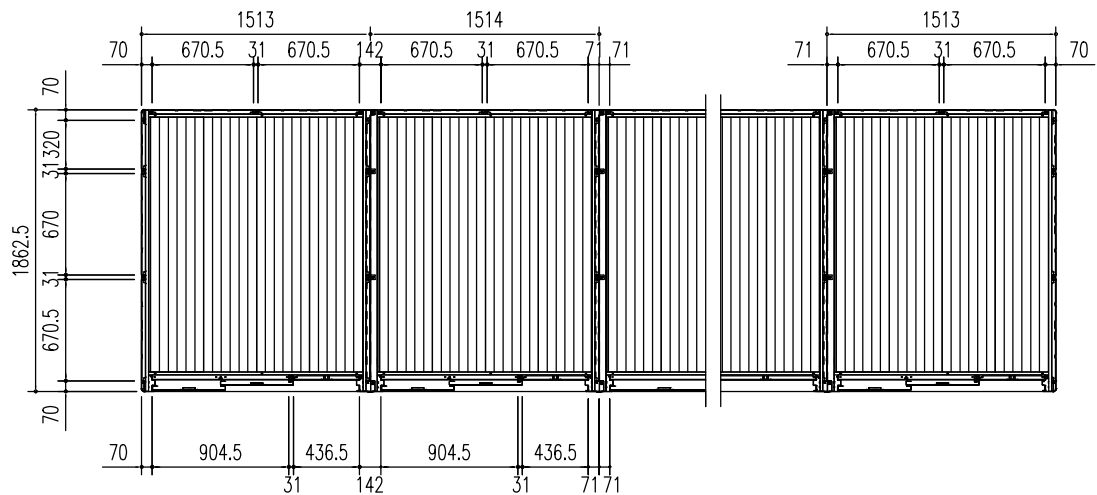
平面図 (S = 1/50)
