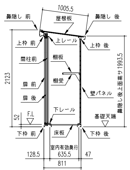
短計図 (S = 1/50)
