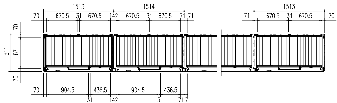
平面図 (S = 1/50)
