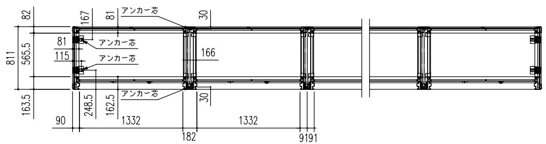
床伏図 (S = 1/50)
