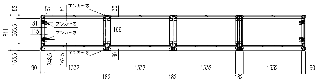
床伏図 (S = 1/50)
