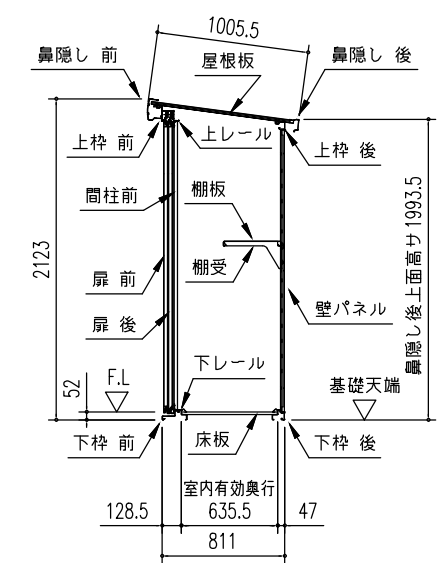
短計図 (S = 1/50)
