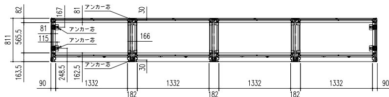
床伏図 (s = 1/50)
