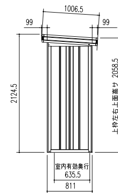
側面立面図 (s = 1/50)
