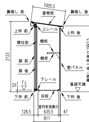
短計図 (s = 1/50)
