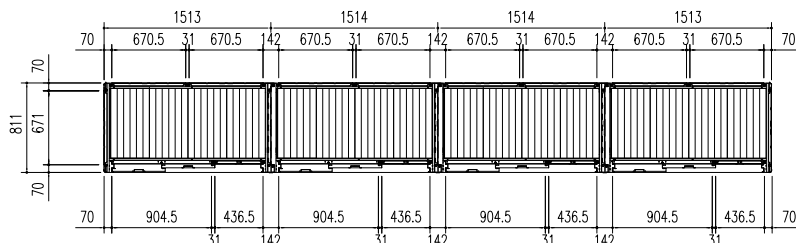
平面図 (s = 1/50)
