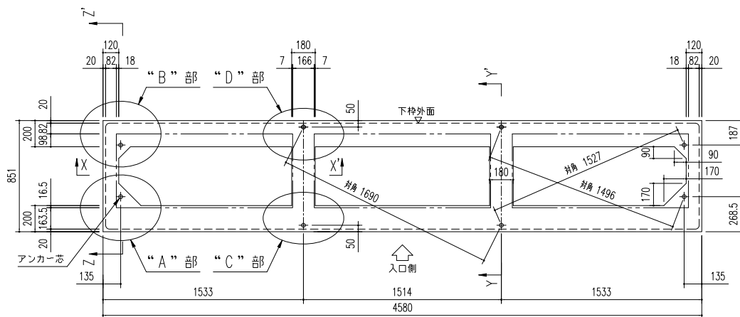
基礎伏図 (S=1/30)
