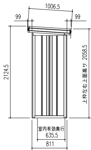
側面立面図 (S = 1/50)
