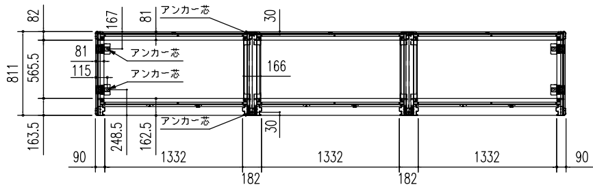
床伏図 (S = 1/50)
