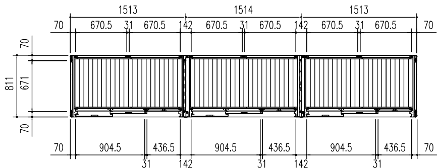
平面図 (S = 1/50)
