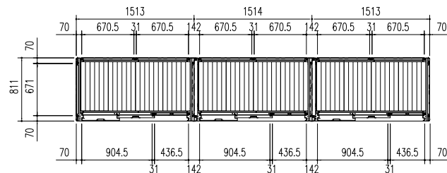
平面図 (S = 1/50)
