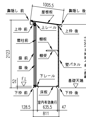
短計図 (S = 1/50)
