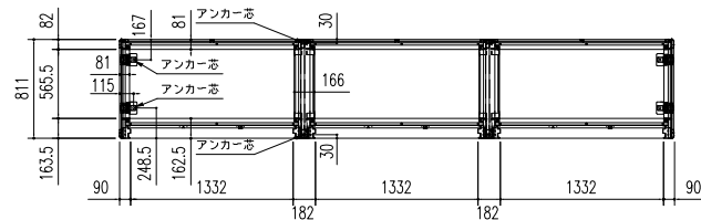
床伏図 (S = 1/50)
