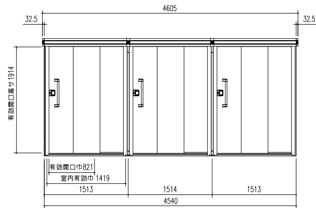
正面立面図 (S = 1/50)
