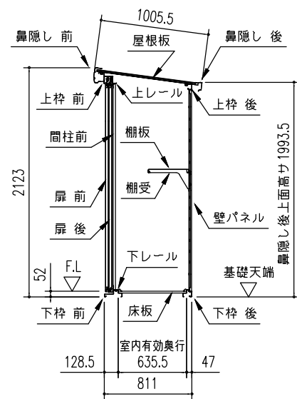
短計図 (S = 1/50)
