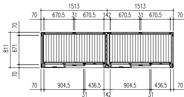
平面図 (S = 1/50)
