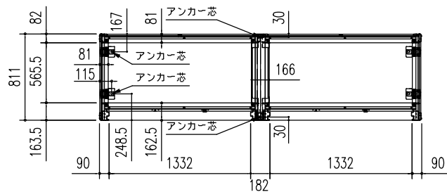
床伏図 (S = 1/50)
