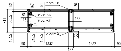
床伏図 (S = 1/50)
