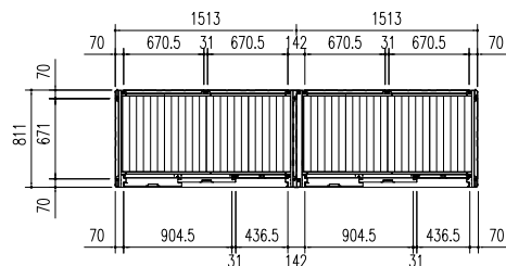
平面図 (S = 1/50)
