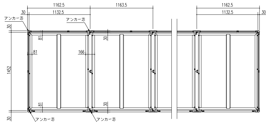
床伏図 (S=1/30)
