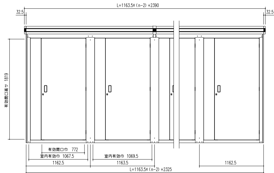
正面立面図 (S=1/30)
