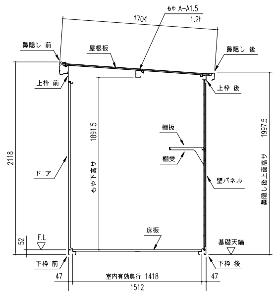
矩計図 (S=1/30)
