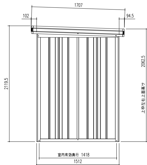
側面立面図 (S=1/30)
