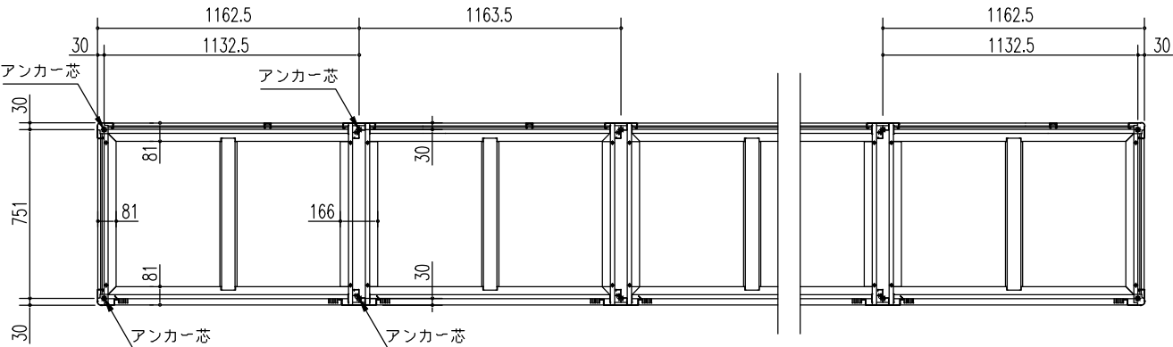
床伏図 (S=1/30)
