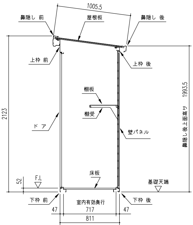
矩計図 (S=1/30)
