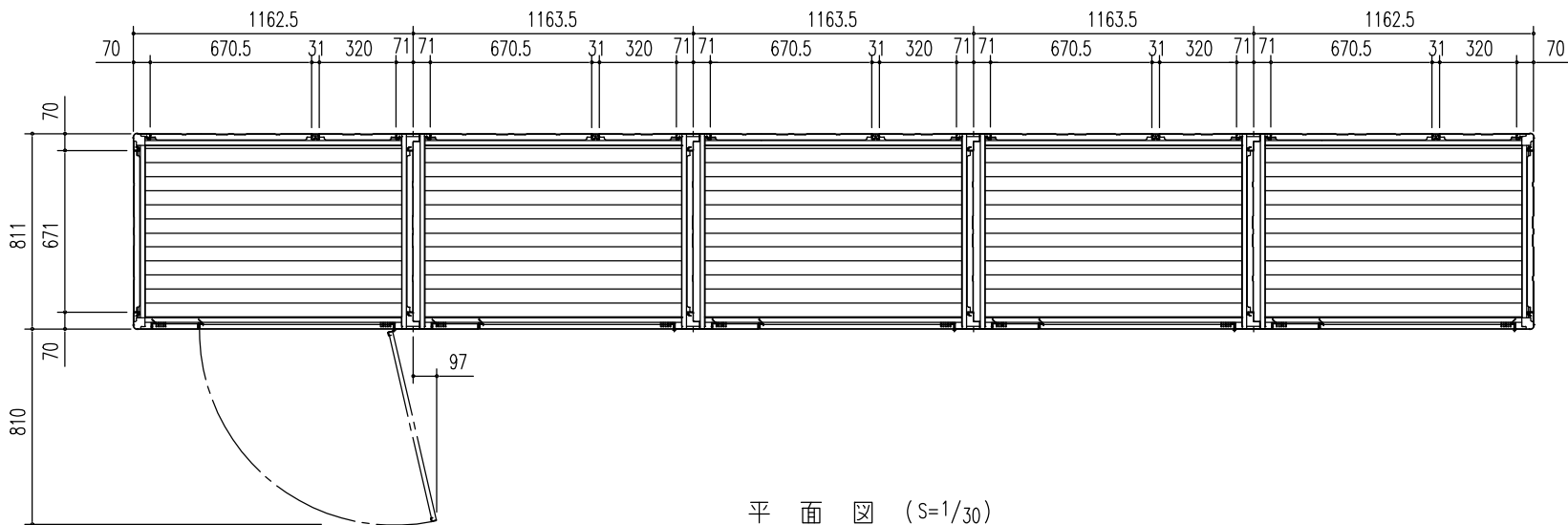
平面図 (S=1/30)
