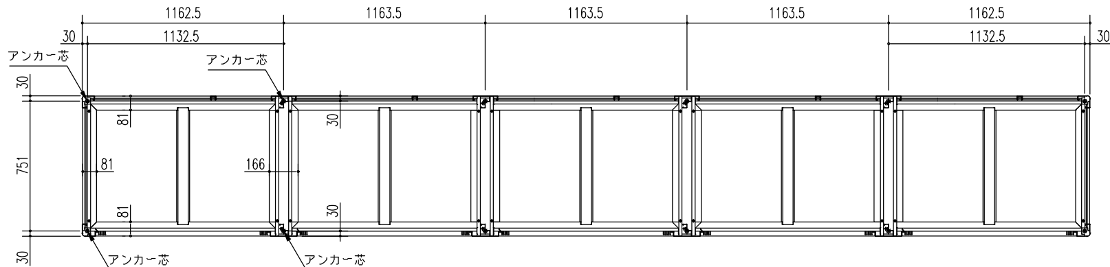
床伏図 (S=1/30)
