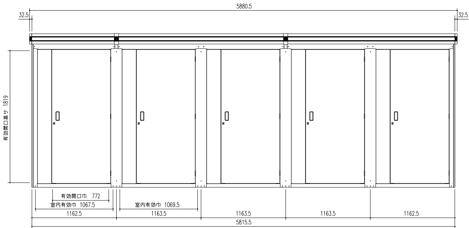
正面立面図 (S = 1/30)
