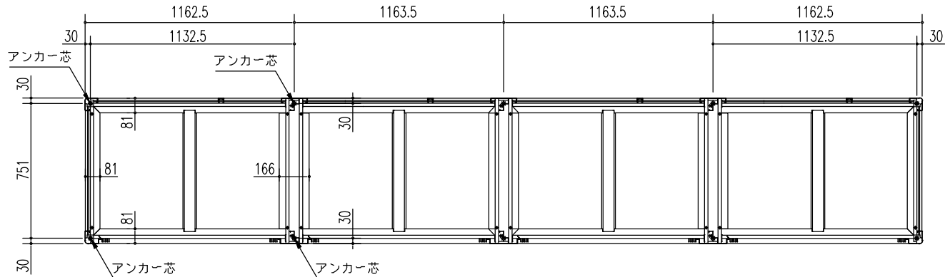
床伏図 (S=1/30)
