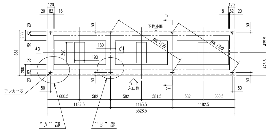
基礎伏図 (S=1/30)
