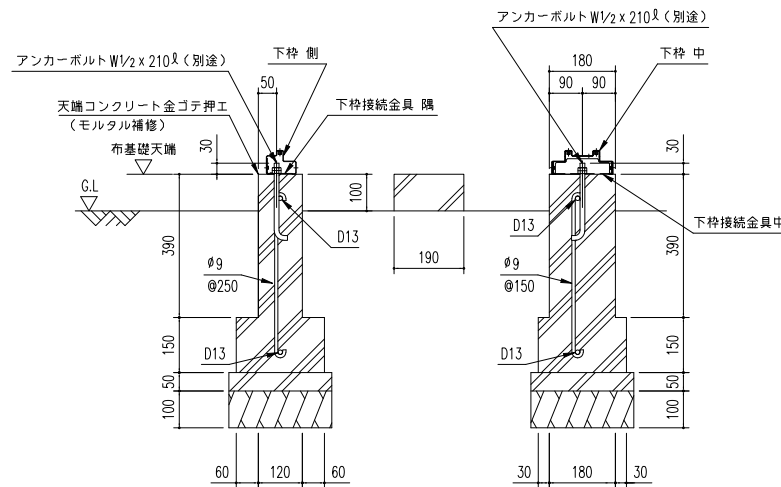
X ~ X' 断面 基礎断面図 (S=1/15)
