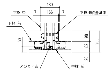
“B” 部詳細図 (S=1/15)
