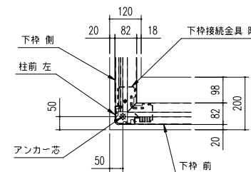
“A” 部詳細図 (S=1/15)
