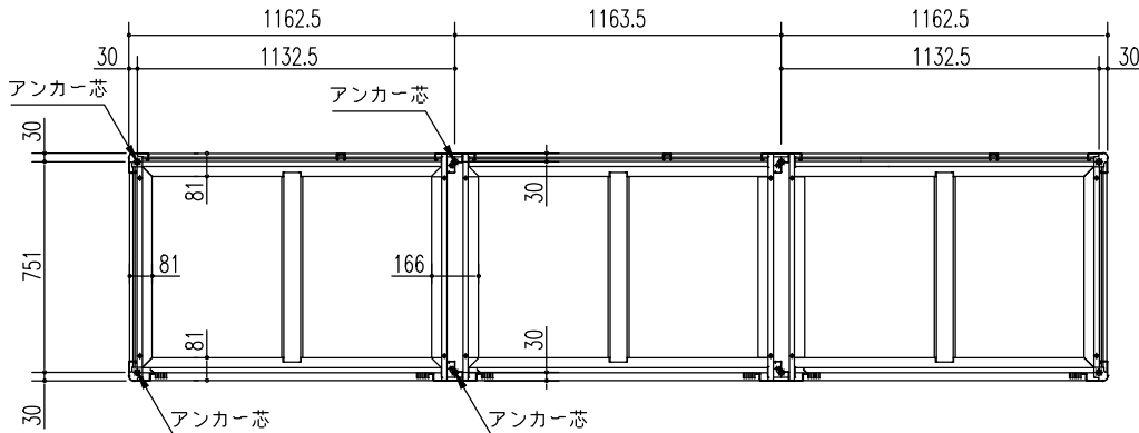
床伏図 (S=1/30)
