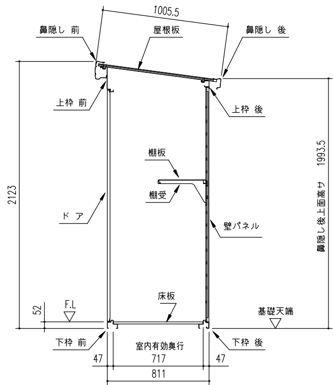
矩計図 (S = 1/30)
