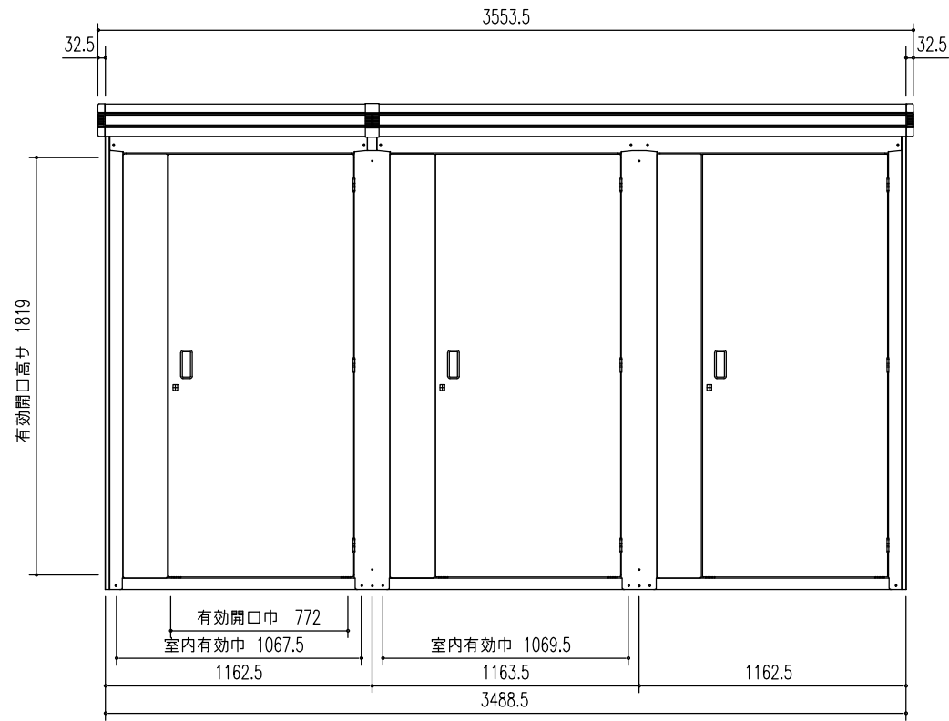
正面立面図 (S = 1/30)
