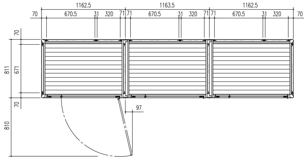
平面図 (S=1/30)
