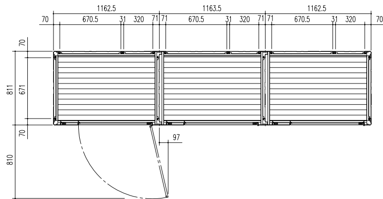
平面図 (S=1/30)
