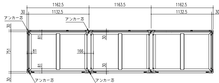
床伏図 (S=1/30)
