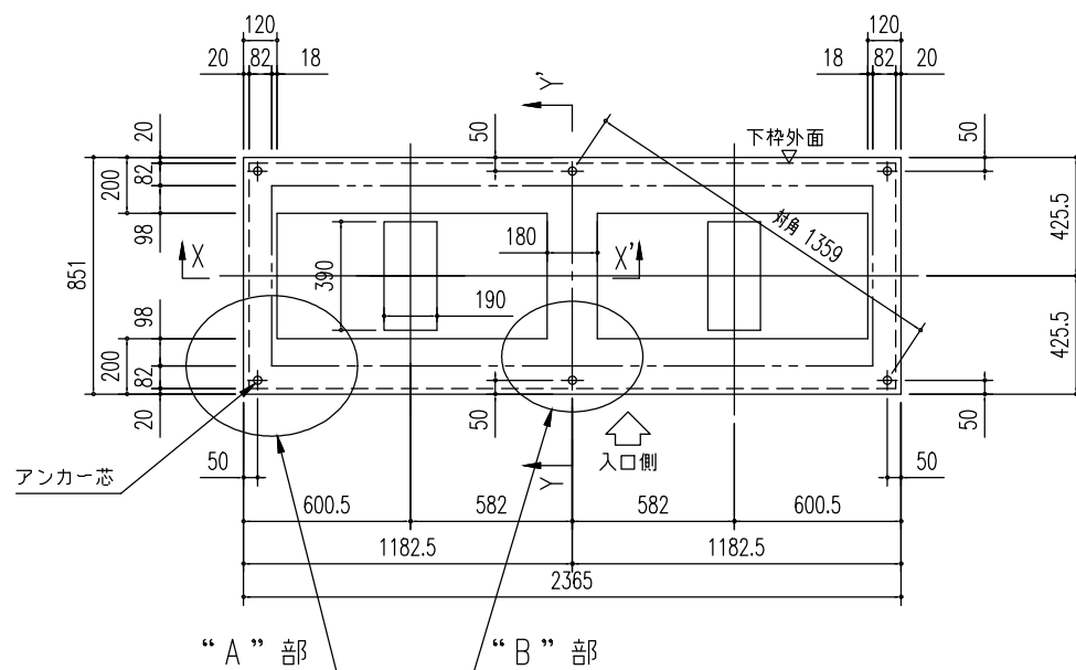
基礎伏図 (S=1/30)
