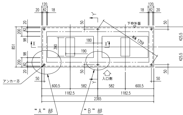
基礎伏図 (S=1/30)
