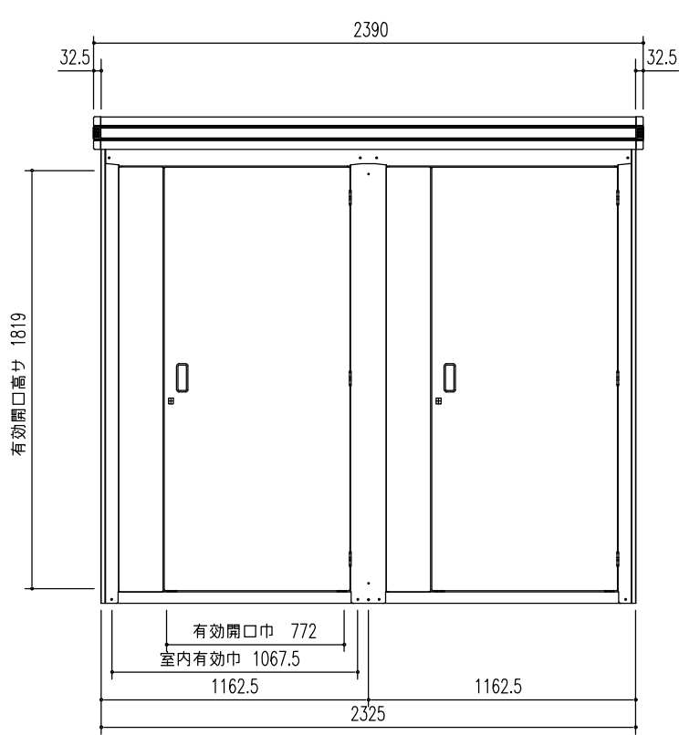
正面立面図 (S = 1/30)
