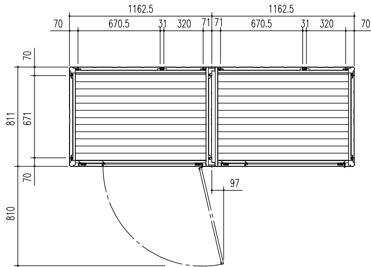
平面図 (S=1/30)
