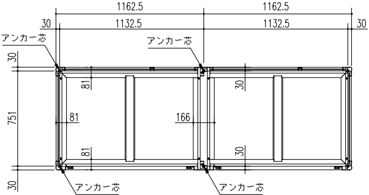
床伏図 (S=1/30)
