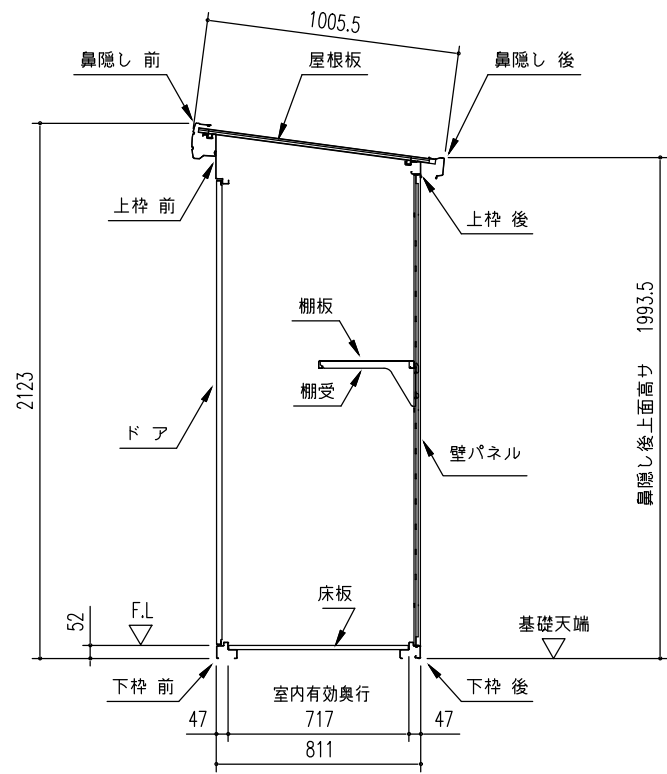
矩計図 (S = 1/30)
