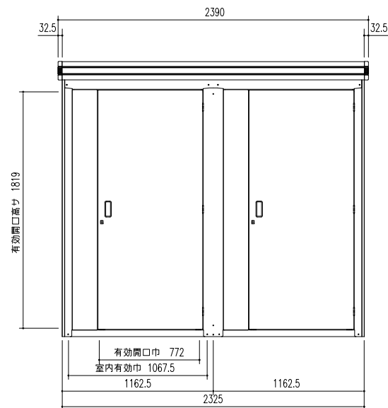
正面立面図 (S=1/30)
