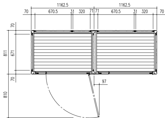
平面図 (S=1/30)
