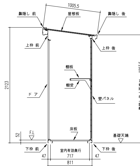
矩計図 (S=1/30)
