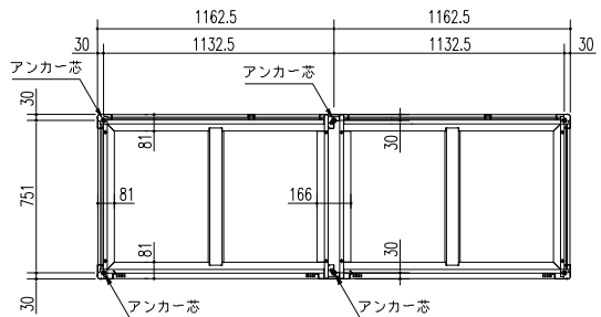
床伏図 (S=1/30)
