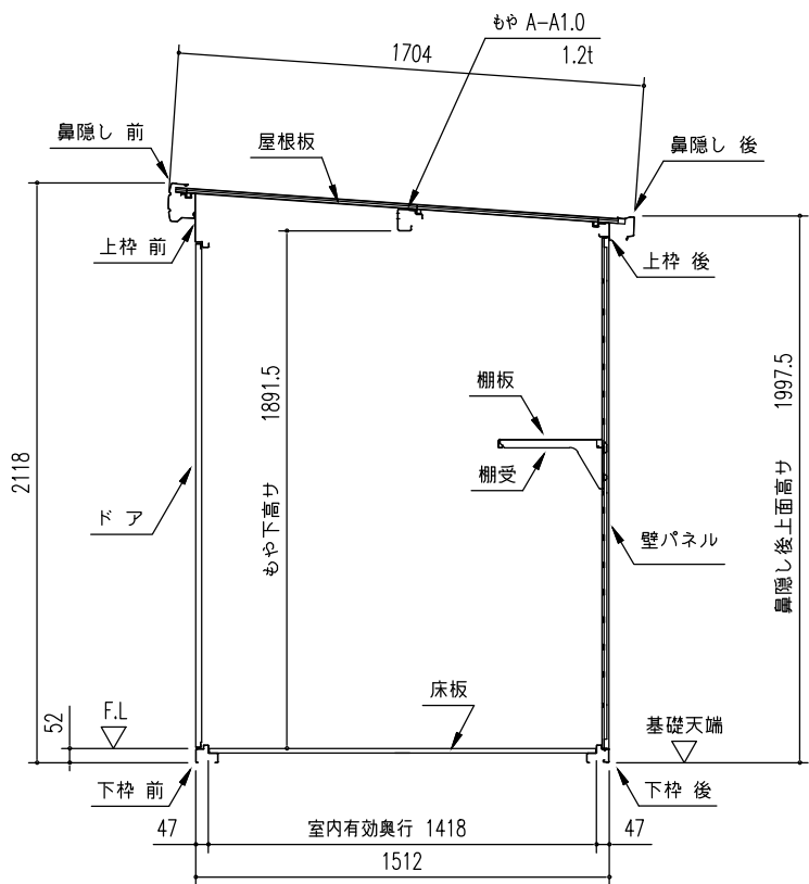
矩 計 図 (S=1/30)
