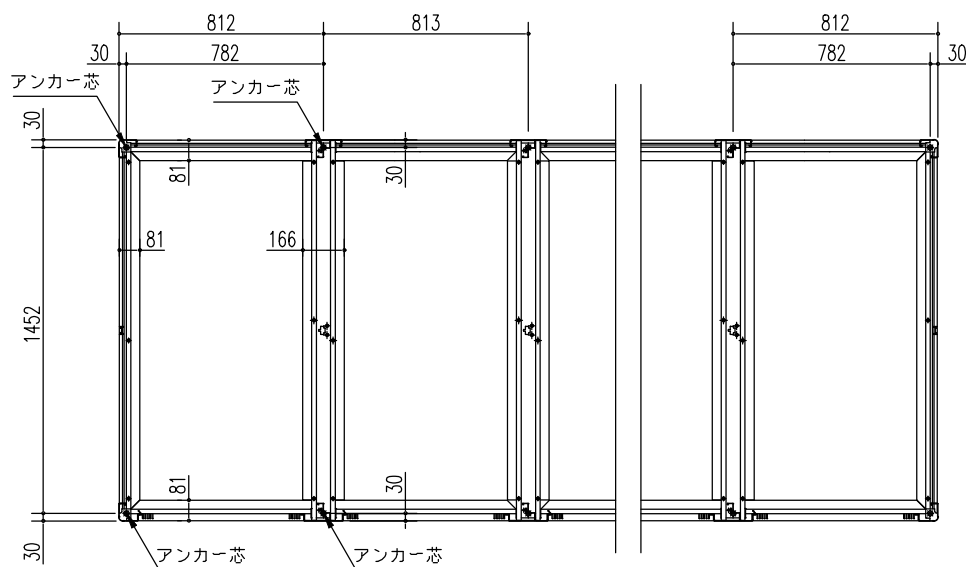
床伏図 (S=1/30)
