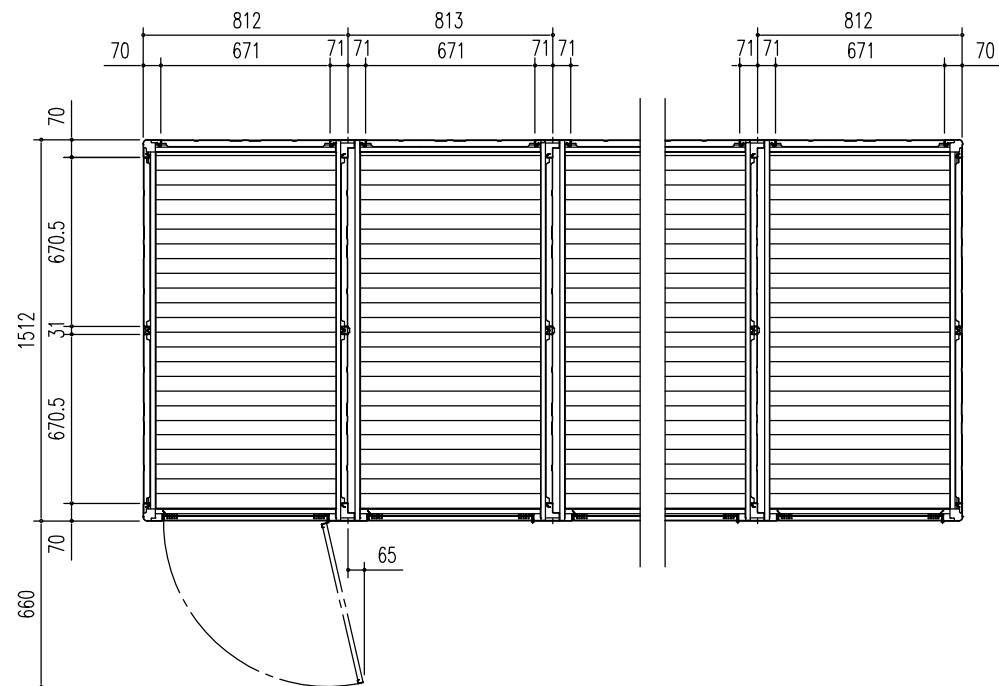
平面図 (S=1/30)
