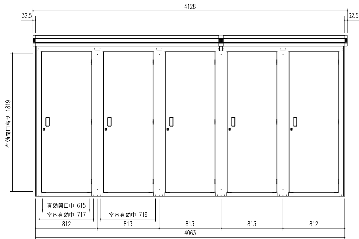
正面立面図 (S=1/30)
