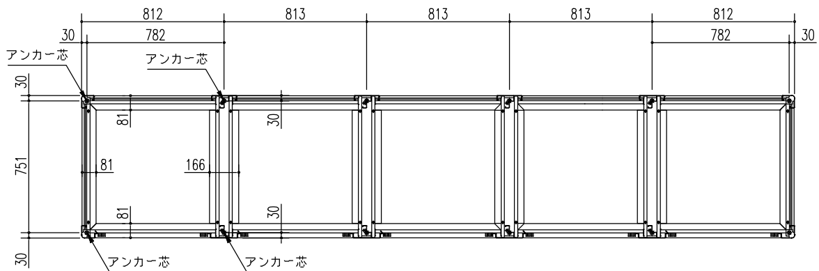
床伏図 (S=1/30)
