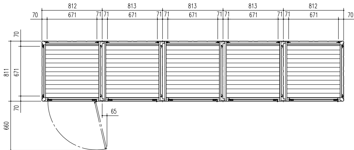
平面図 (S=1/30)
