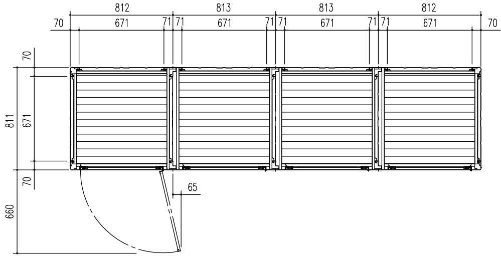
平面図 (S=1/30)
