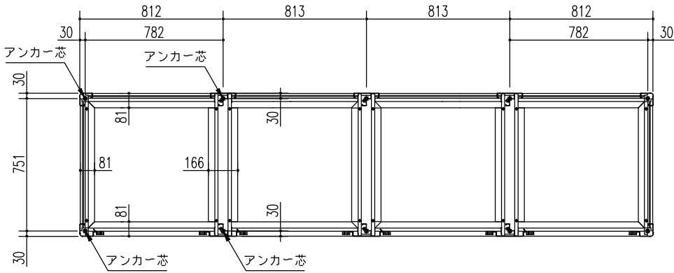
床伏図 (S=1/30)
