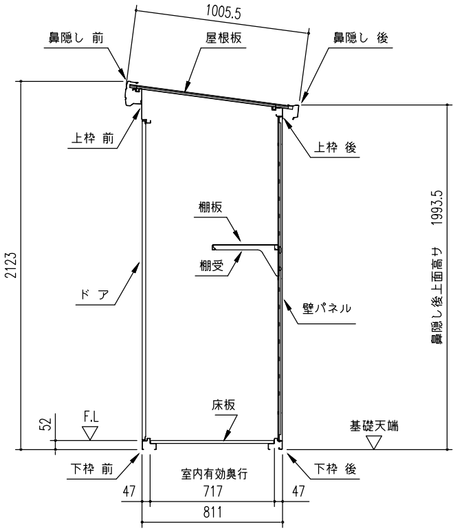
矩 計 図 (S = 1/30)
