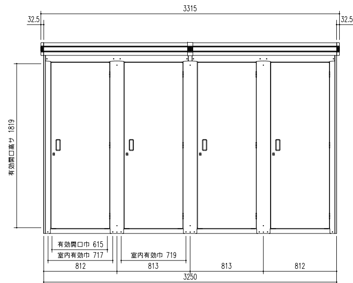
正面立面図 (S=1/30)
