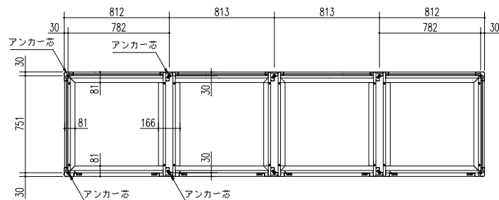
床伏図 (S=1/30)
