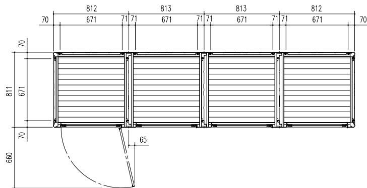
平面図 (S=1/30)
