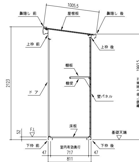
矩計図 (S=1/30)
