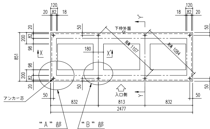
基礎伏図 (S=1/30)
