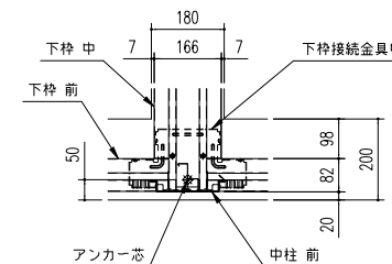
“B” 部詳細図 (S=1/15)
