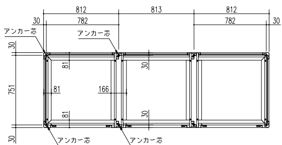
床伏図 (S = 1/30)
