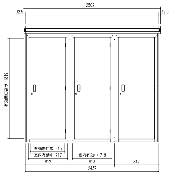
正面立面図 (S = 1/30)
