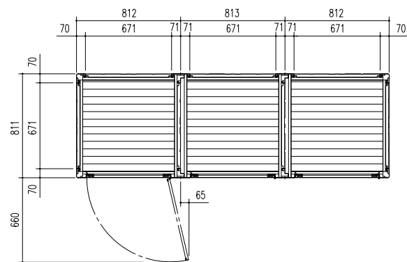
平面図 (S = 1/30)
