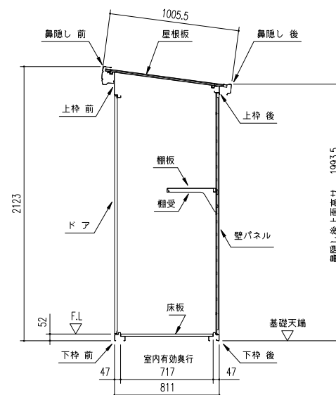
矩計図 (S = 1/30)
