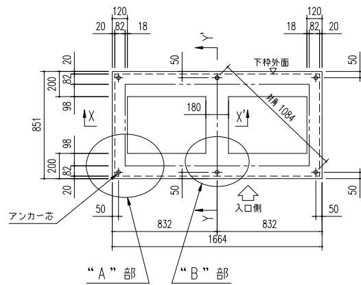
基礎伏図 (S=1/30)
