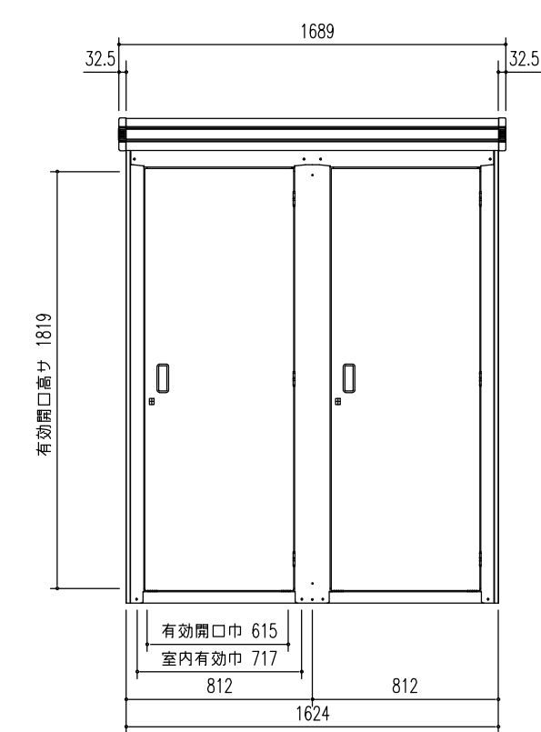
正面立面図 (S = 1/30)
