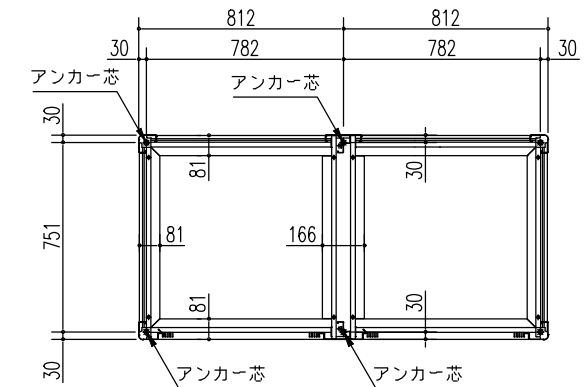
床伏図 (S = 1/30)
