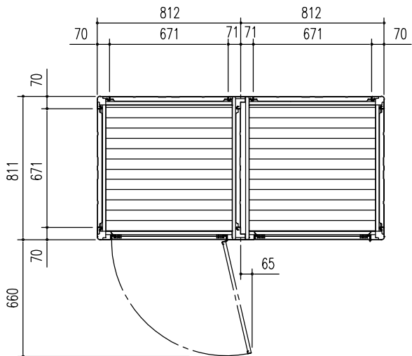
平面図 (S = 1/30)
