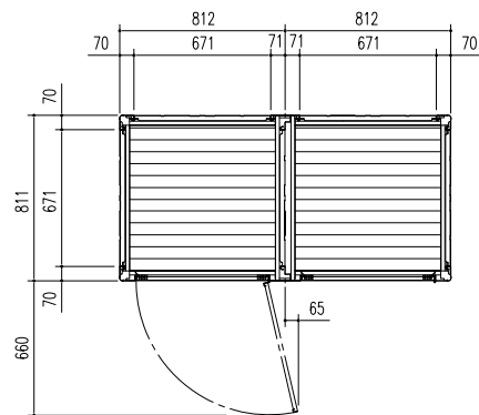
平面図 (S=1/30)
