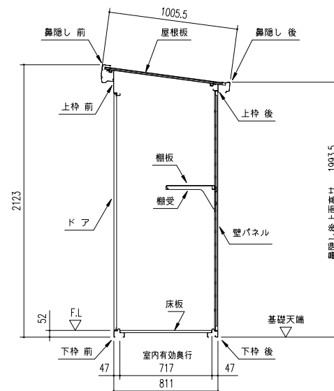
矩計図 (S=1/30)
