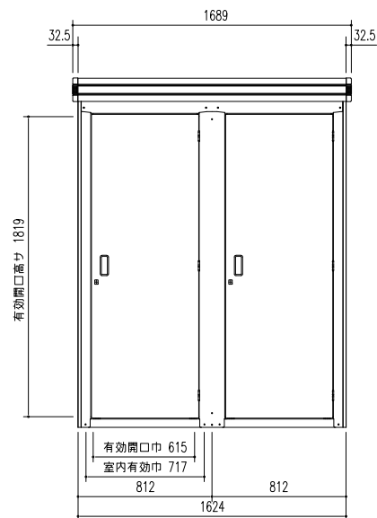
正面立面図 (S=1/30)
