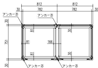
床伏図 (S=1/30)
