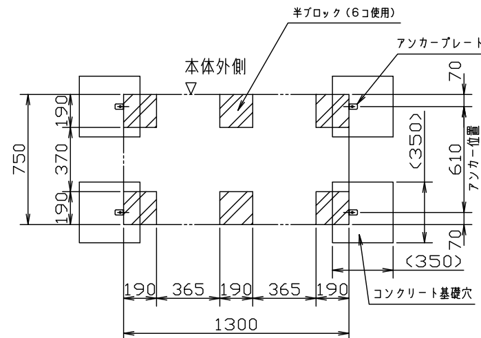
<半ブロック配置参考図>
