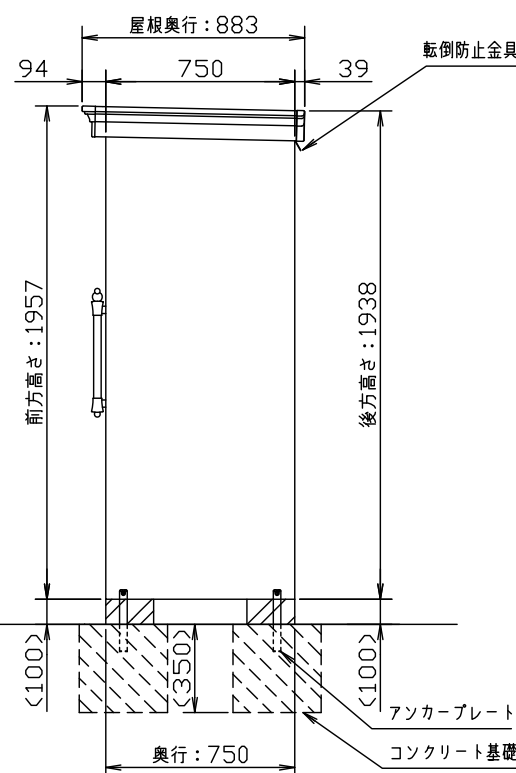
<側面立面図 S=1/30>
