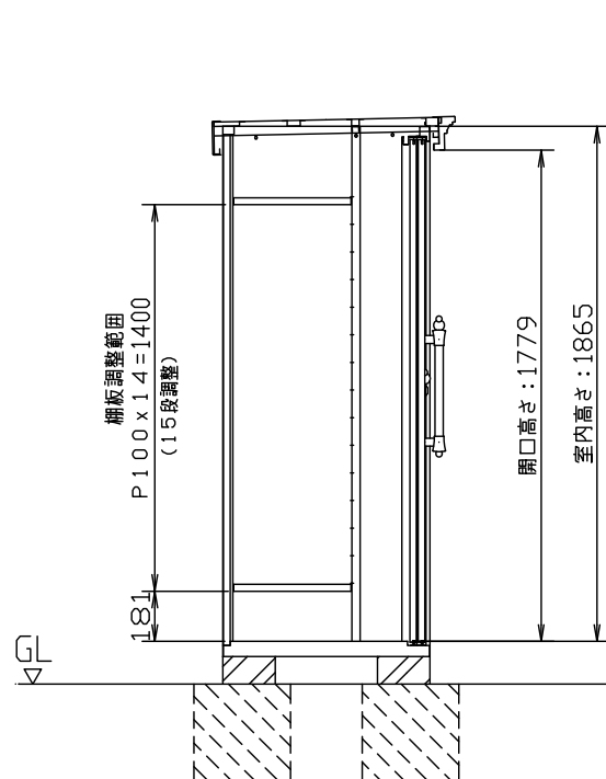
<矩計図 S=1/30>
