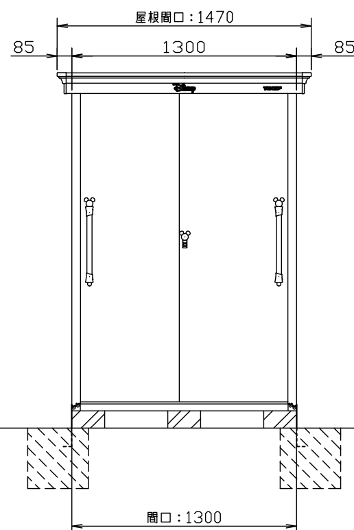
<正面立面図 S=1/30>
