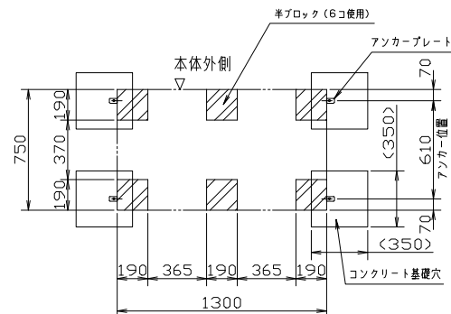
<半ブロック配置参考図>
