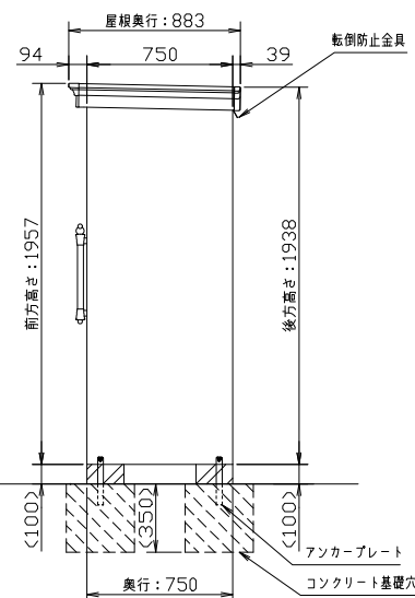
<側面立面図 -S=1/30>
