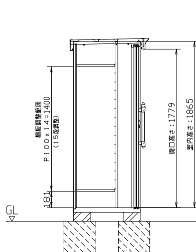
<矩計図 S=1/30>
