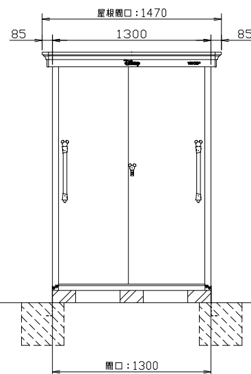
<正面立面図 -S=1/30>
