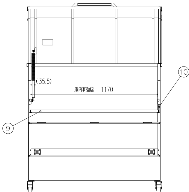
正面立面図（フタ・前扉オープン）
