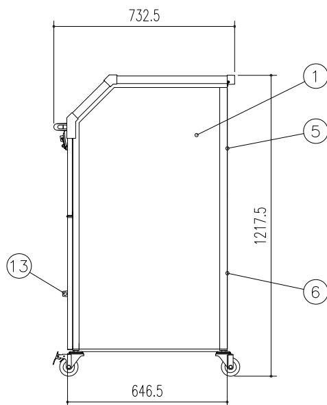
側面立面図
