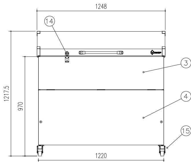
正面立面図
